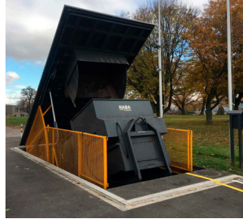
HABA MEGA S-contenedor compactador residuos soterrado
